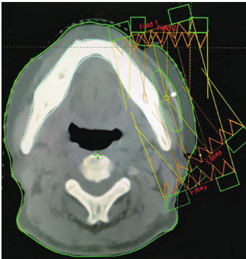
图 4 下颌外侧靶区放疗计划的切线对穿野设计
