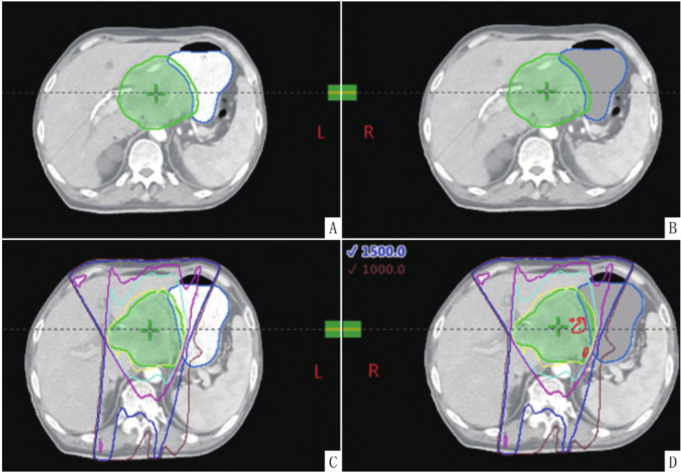
注：A. 定位时胃内大量高密度造影剂分布图像；B. 采用水密度填充替代造影剂后的胃部 CT 图像；C. 未做造影剂水替换的原计划设计；D. 把未改变造影剂密度的计划复制到替代密度的 CT 图像上，在相同的照射野和机器跳数情况下，靶区内会出现高剂量区域（红线所示），可能会导致胃壁的高剂量照射。
